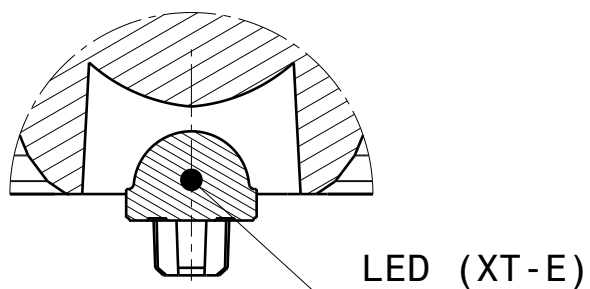
Detail B Scale: 5:1
